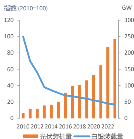
光伏装机与电池白银装载量*
